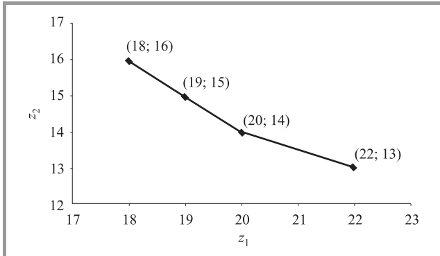
Fig. 6. Pareto front.
