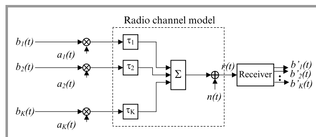
Fig. 1. DS-CDMA model.
