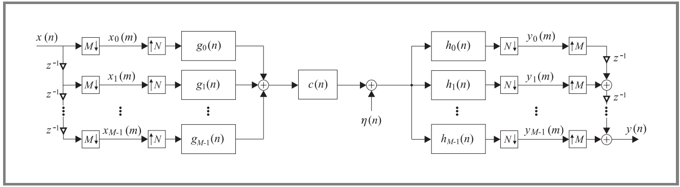
Fig. 1. Redundant precoder.
